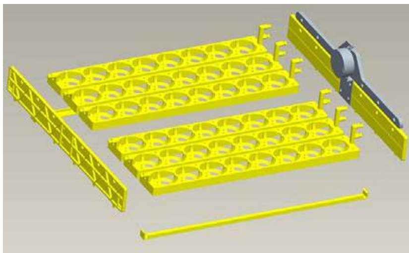
Рисунок 3. Соберите лотки для яиц: соедините каждый лоток с блоком поворота. Закрепите боковые стенки с помощью планок.
